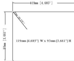
Cutout Dimensions
