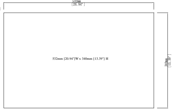
Cutout Dimensions
