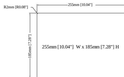
Cutout Dimensions
