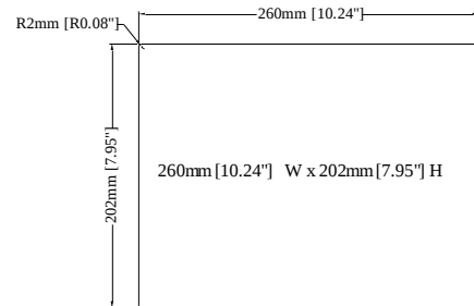
Cutout Dimensions
