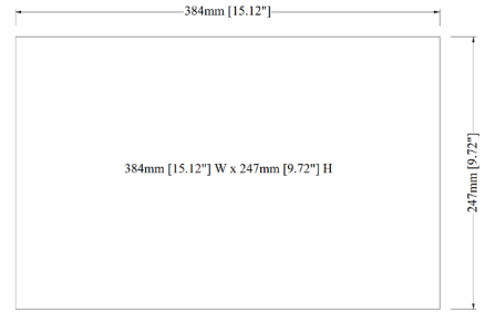
Cutout Dimensions
